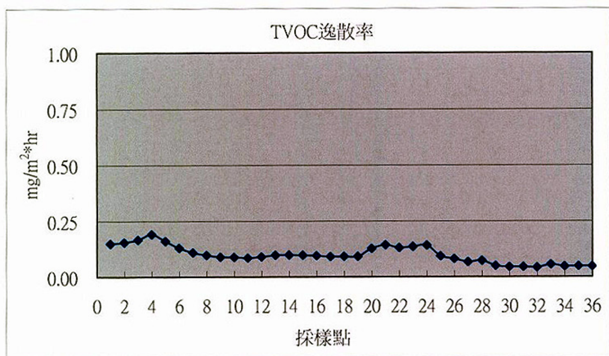
Fig1. 建材中總揮發性有機物逸散率
